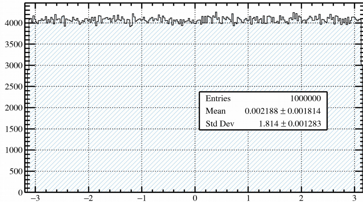
\phi Gottfried-Jackson Frame \phi
