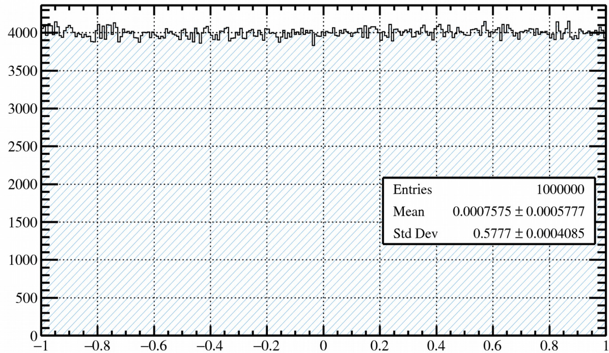
\phi Gottfried-Jackson Frame \cos(\theta)
