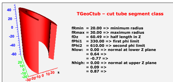
Figure 18-13 TGeoCtub Class
